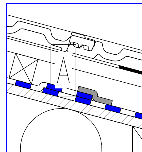
zakłady membrany paroprzepuszczalnej uszczelnione taśmą SIGA Wigluv
